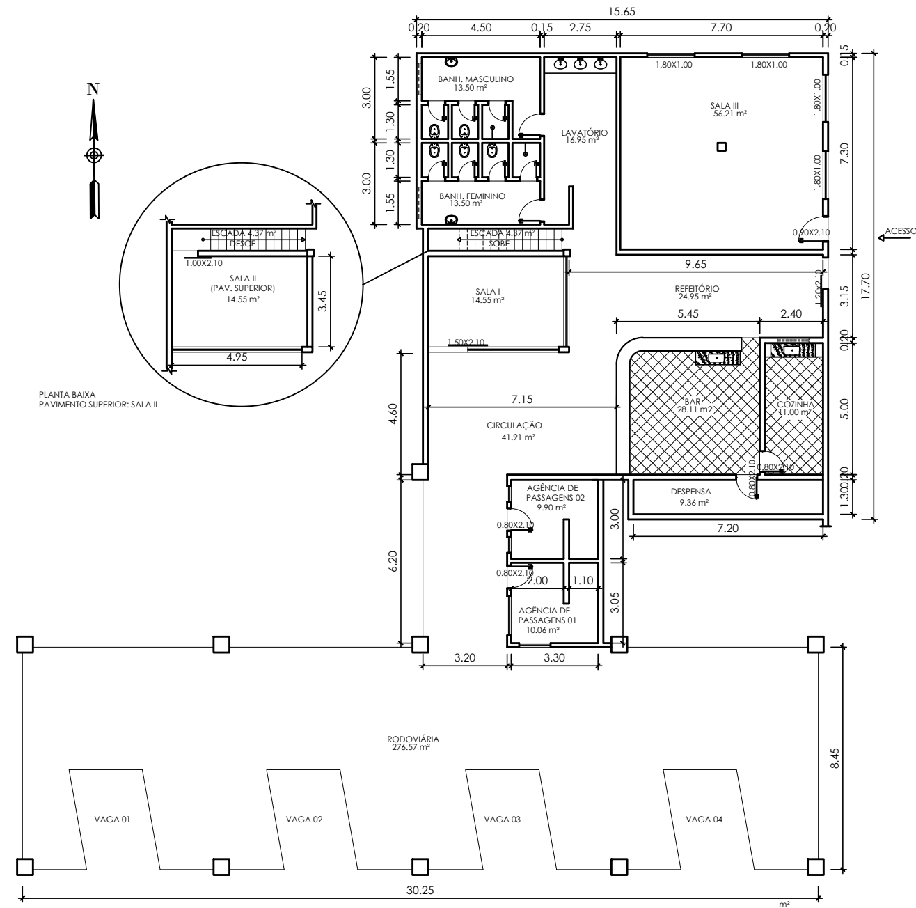
PLANTA BAIXA TÉRREO ESCALA 1/200
